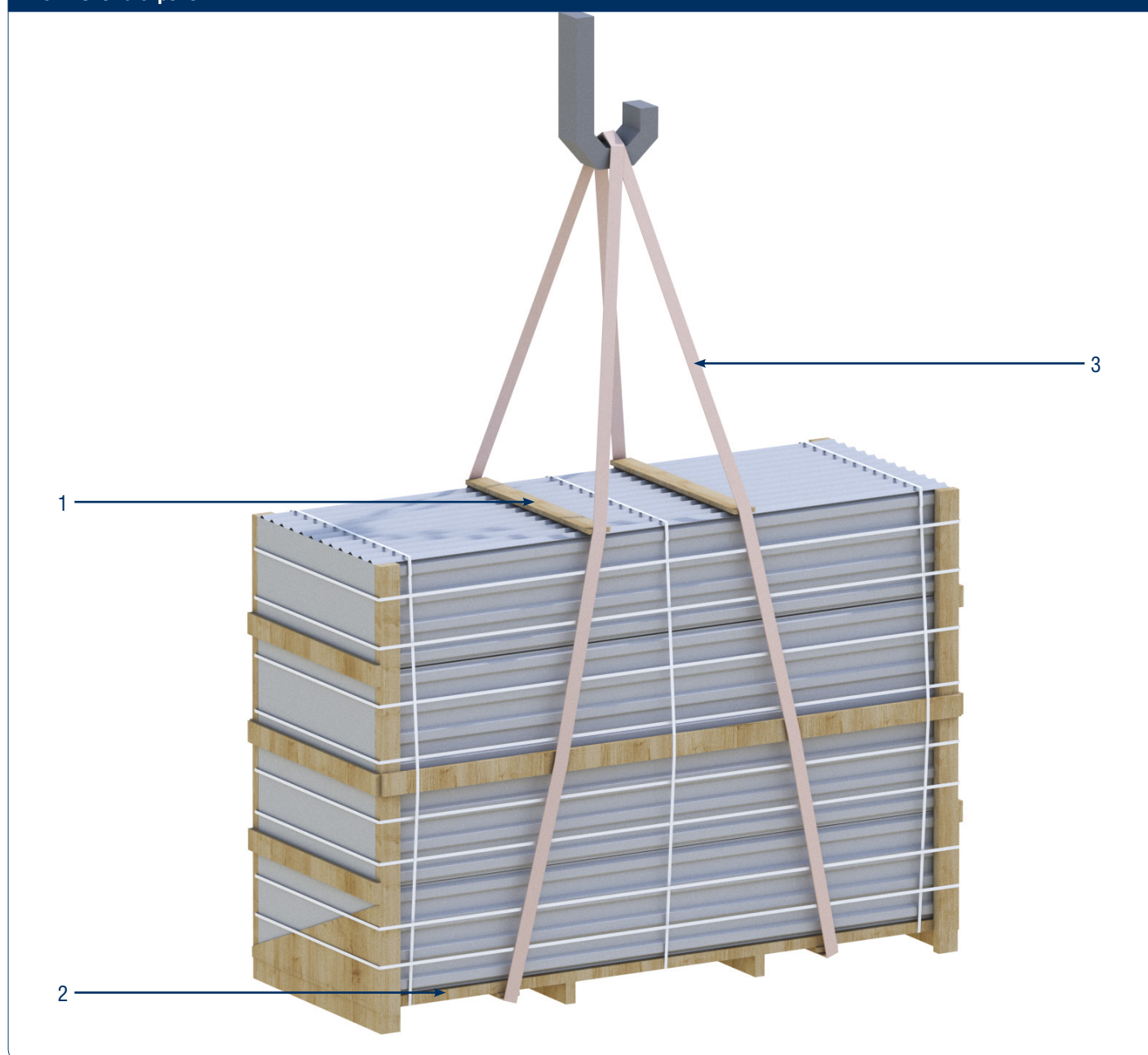
Рис. 1. Схема строповки
